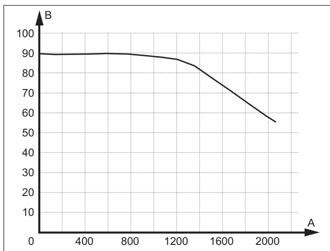
A Көлемдік ағын, л/сағ B Қалдық беру қысымы, кПа
