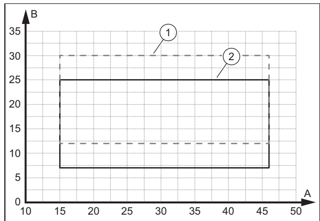
A Temperatură exterioară B Temperatura agentului termic 1 Limite de aplicabilitate, faza de pornire a răcirii 2 Limite de aplicabilitate, regim normal de funcționare a răcirii
