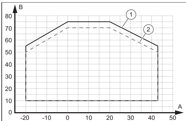
A Temperatură exterioară B Temperatura agentului termic 1 Limite de aplicabilitate, regim normal de funcționare pentru apa caldă menajeră 2 Limite de aplicabilitate, faza de pornire a apei calde menajere
