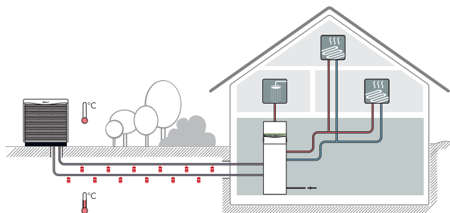
Prepojenie tepelného čerpadla flexoCOMPACT exclusive s jeho vonkajšou vzduchovou jednotkou.
